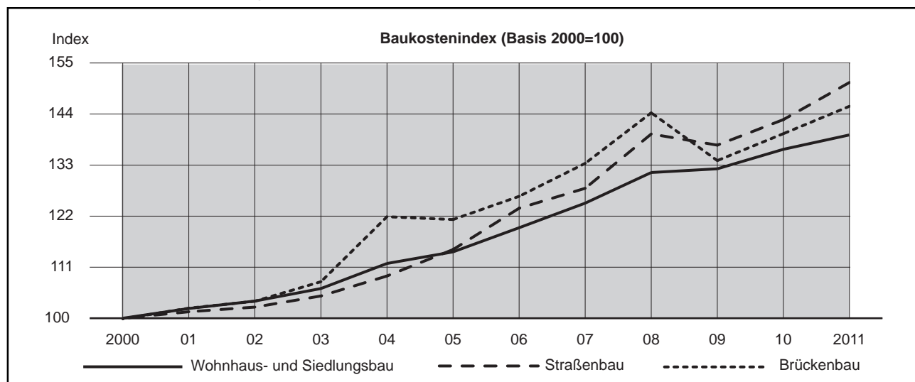
Grafik 11.2 Entwicklung des Baukostenindex
