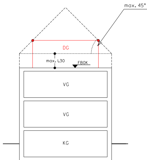
Schnitt
