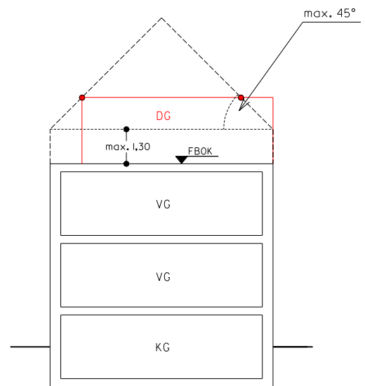
Schnitt 1
