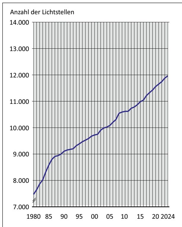
Grafik 12.6 Öffentliche Beleuchtung
