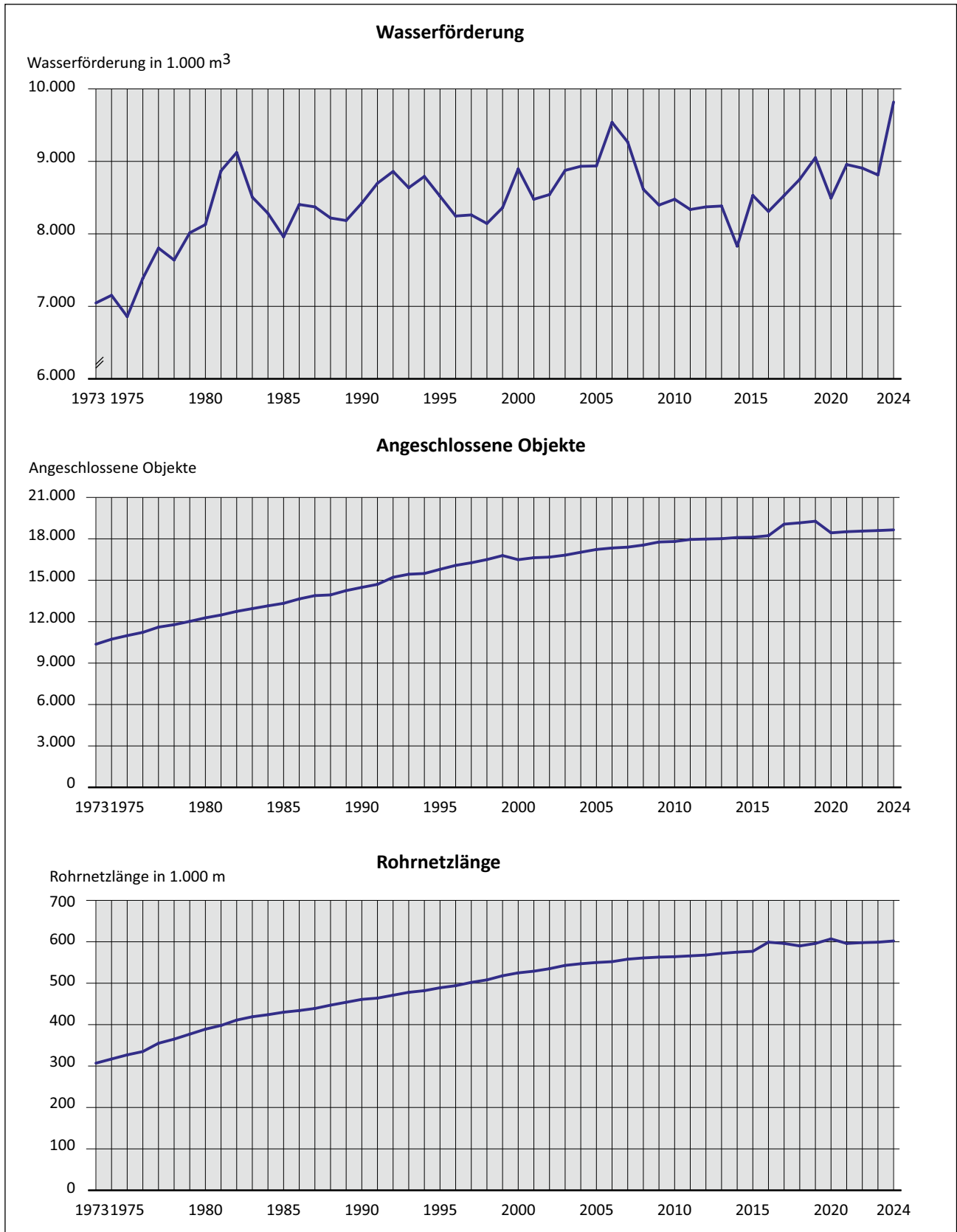
Grafik 17.2 Wasserversorgung
