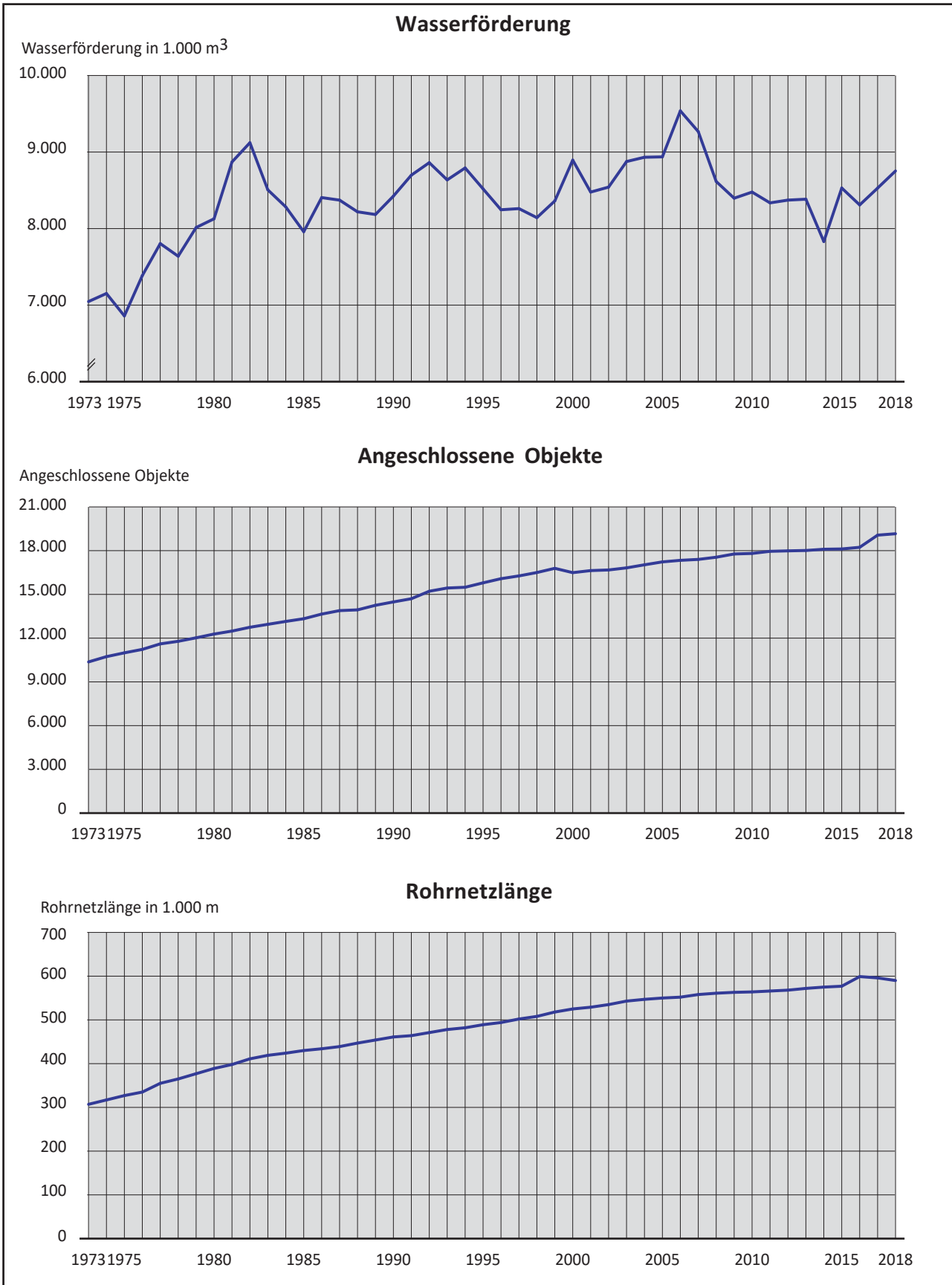
Grafik 17.2 Wasserversorgung
