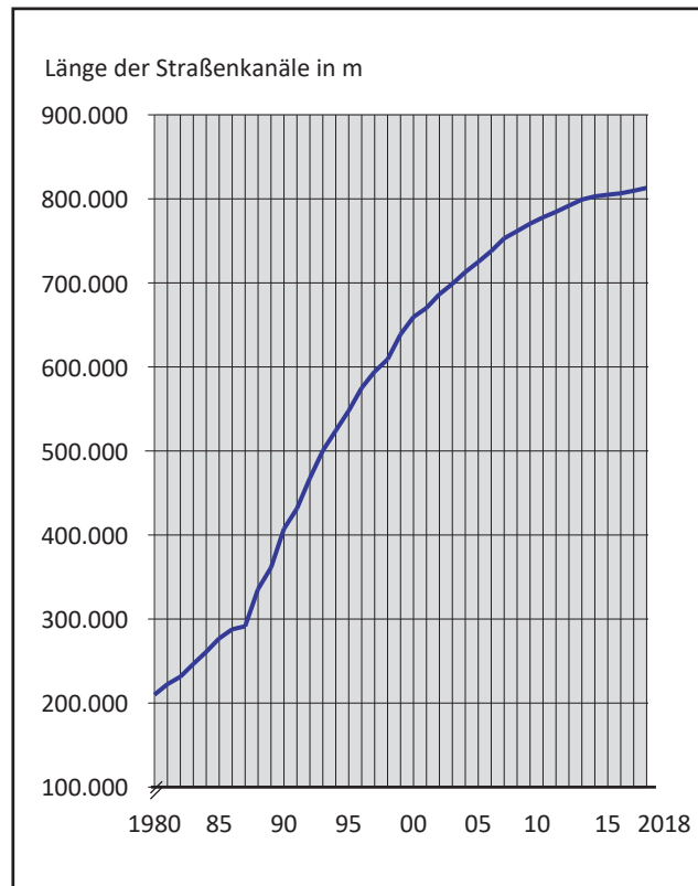
Grafik 12.5 Kanalisation
