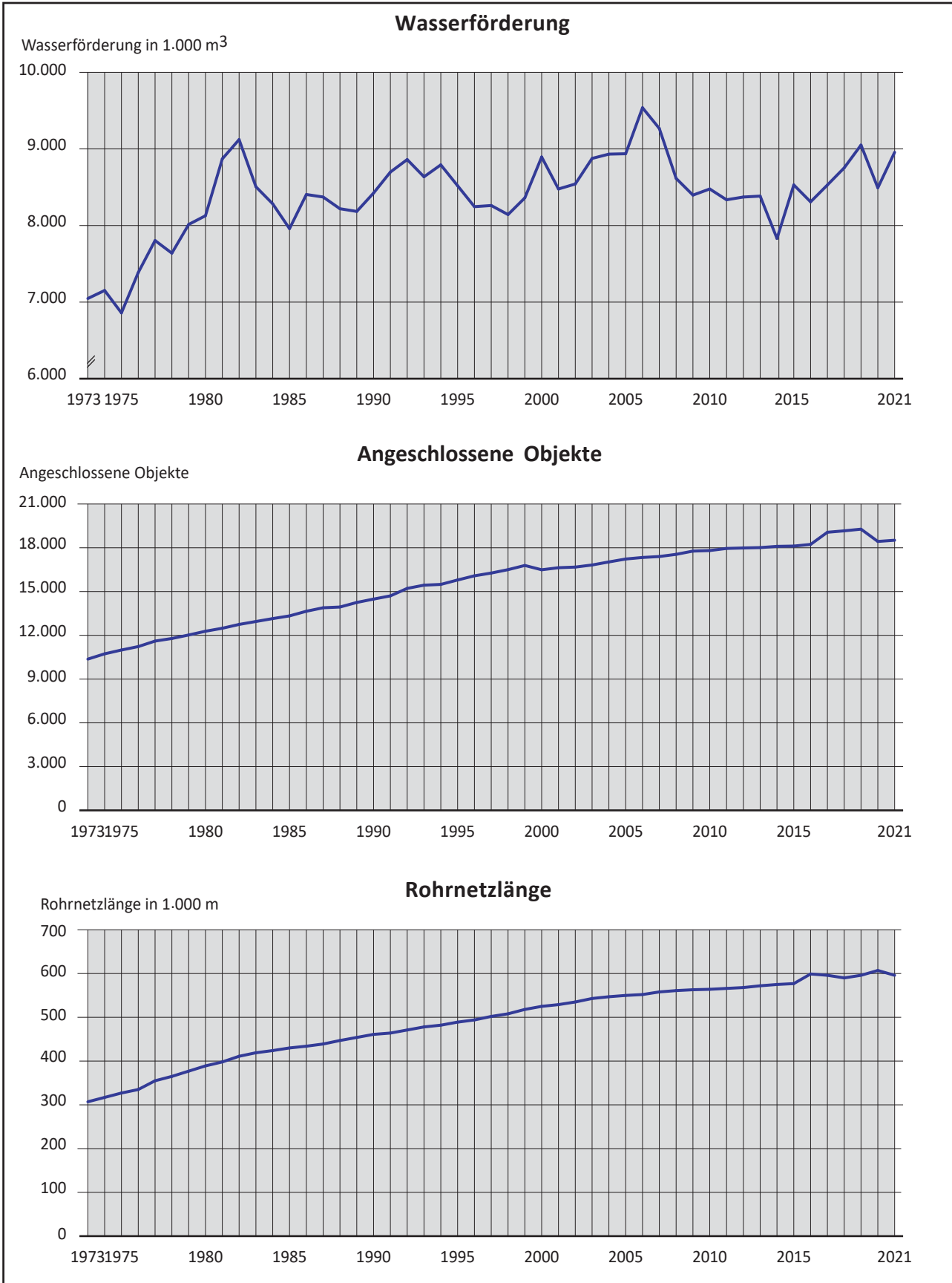
Grafik 17.2 Wasserversorgung
